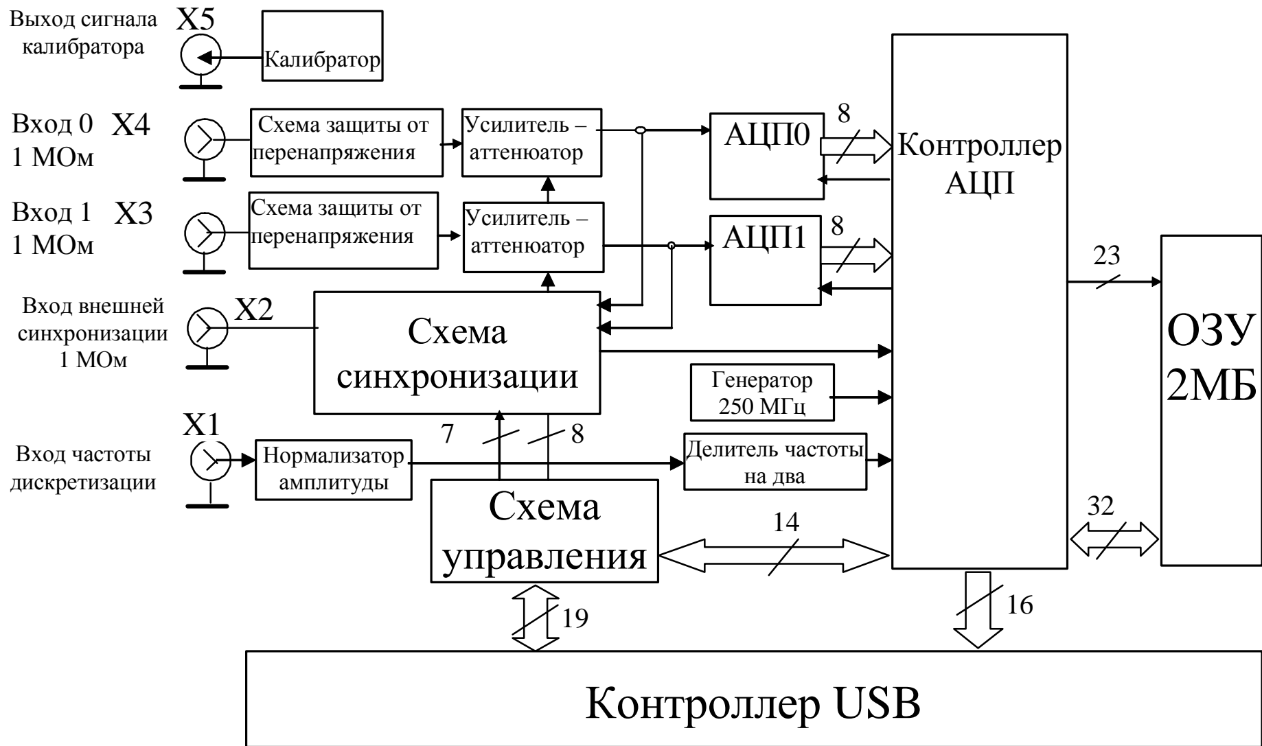
Рис. 1 Функциональная схема ЛА-н4USB
