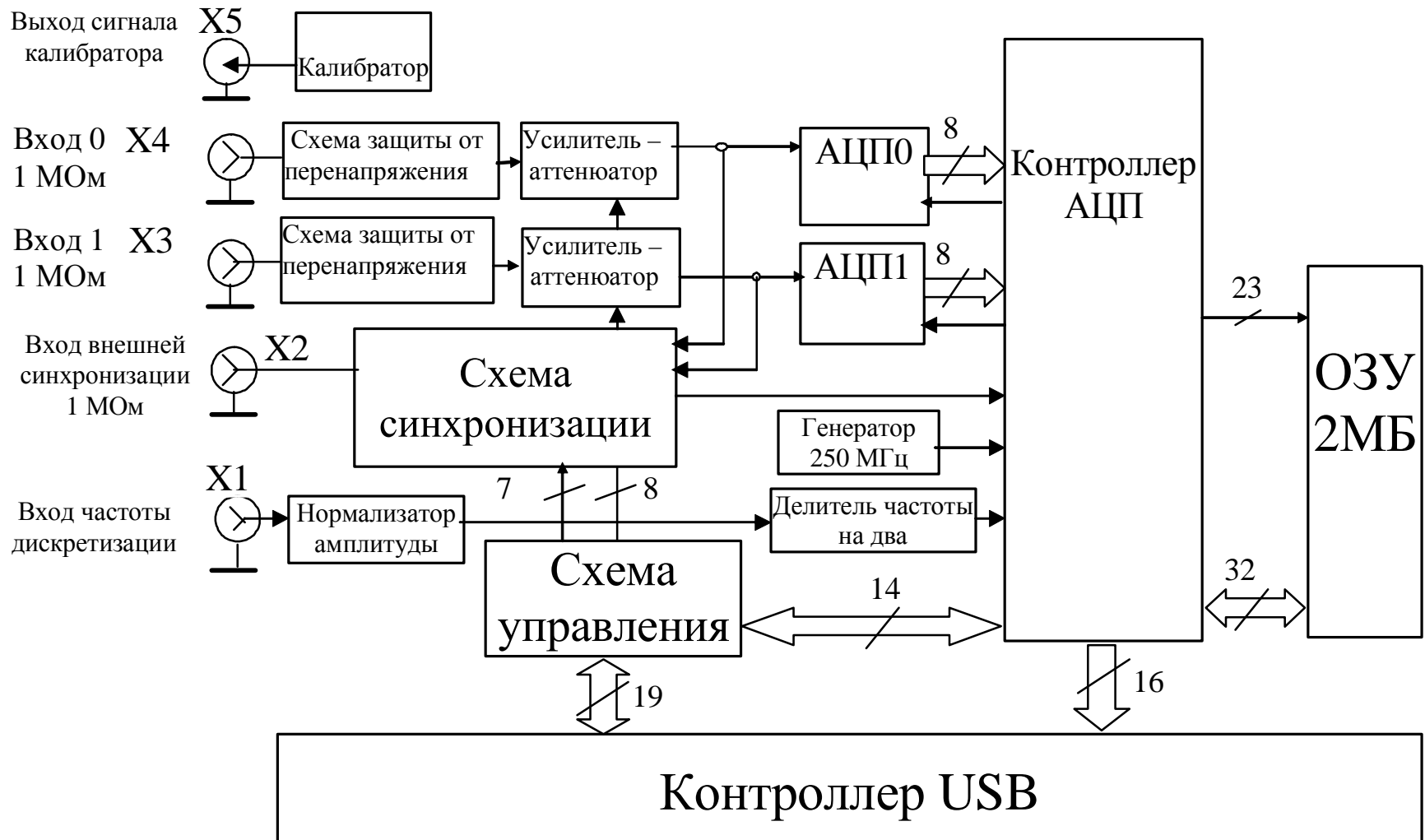
Рис. 1.1 Функциональная схема ОЦЗС-02(250USB)-2/4/6/8
